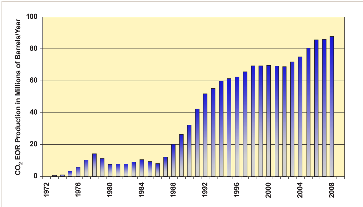
U.S. CO 2 EOR Production
